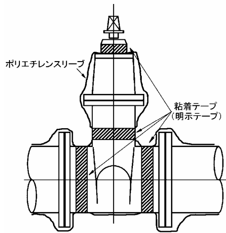
仕切弁部
