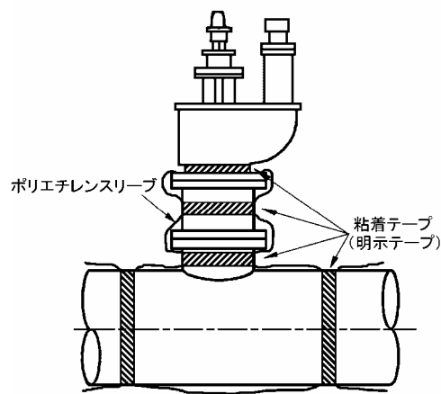
消火栓部
