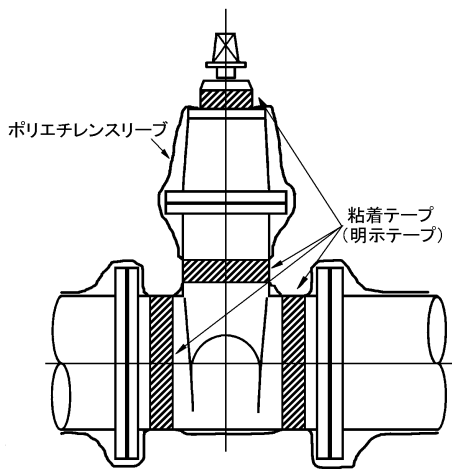
仕切弁部
