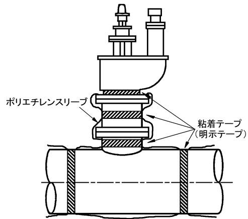
消火栓部
